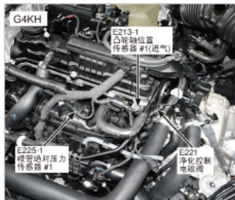
32. 发动机左侧
