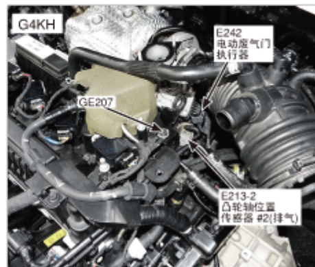
33. 发动机后部
