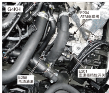
35. 变速器顶部
